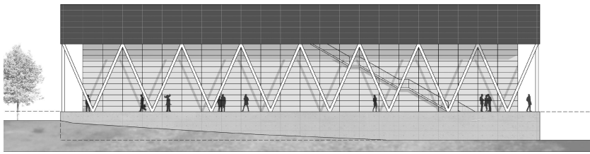
ansicht süd
