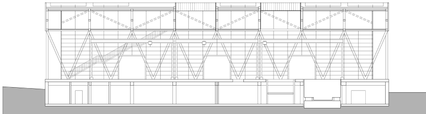
längsschnitt
