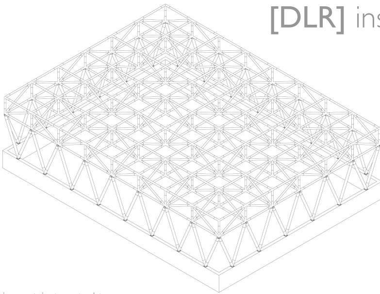
isometrie tragstruktur
